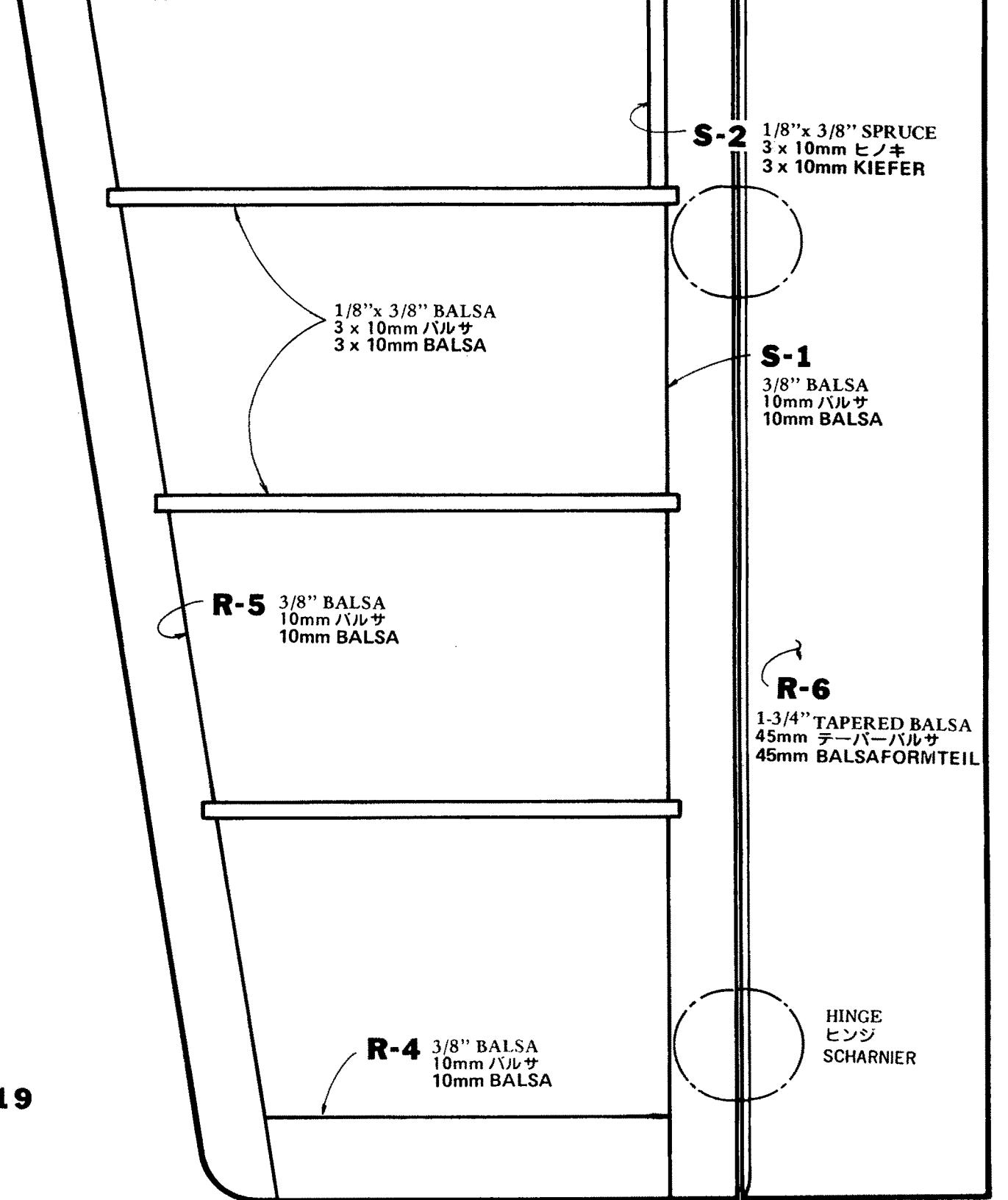
STABILIZER TOP VIEW 尾翼平面図 HÖHENRUDER VON OBEN
