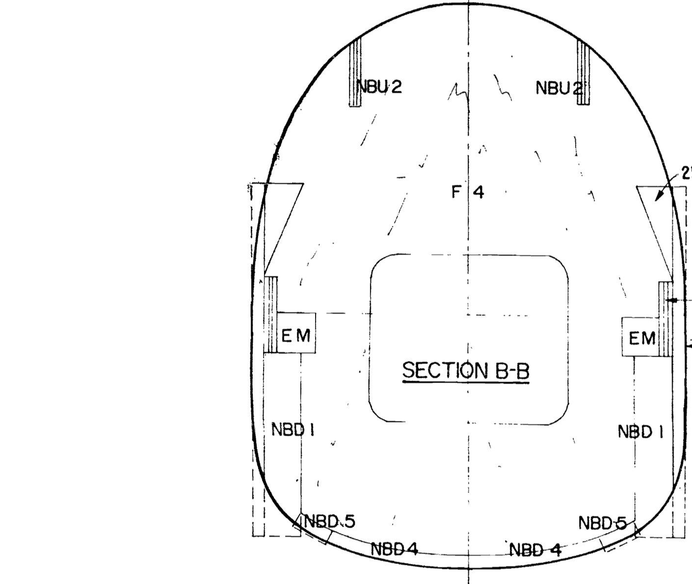
側板補強
