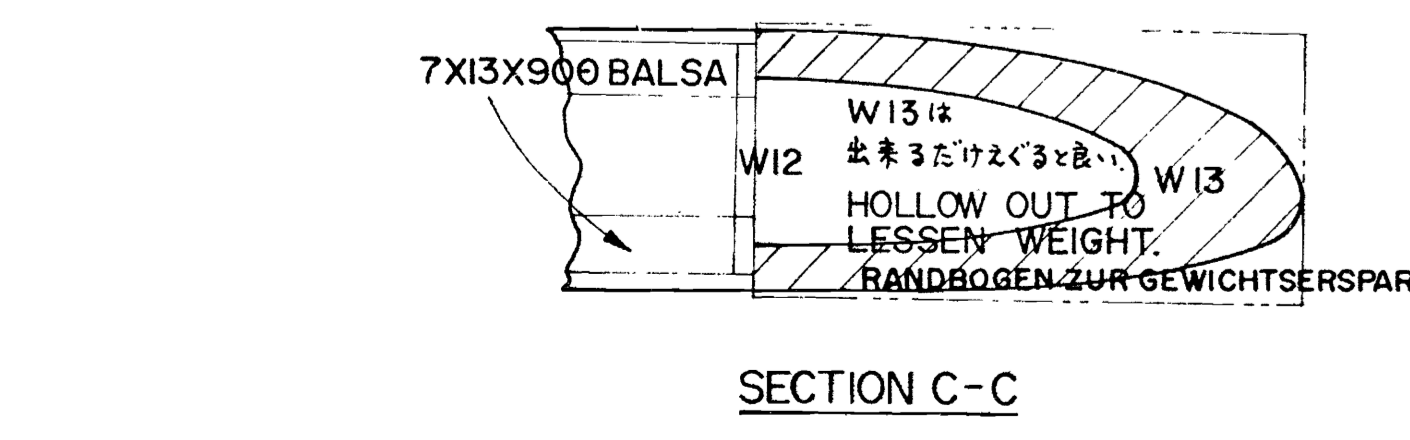
側板補強
