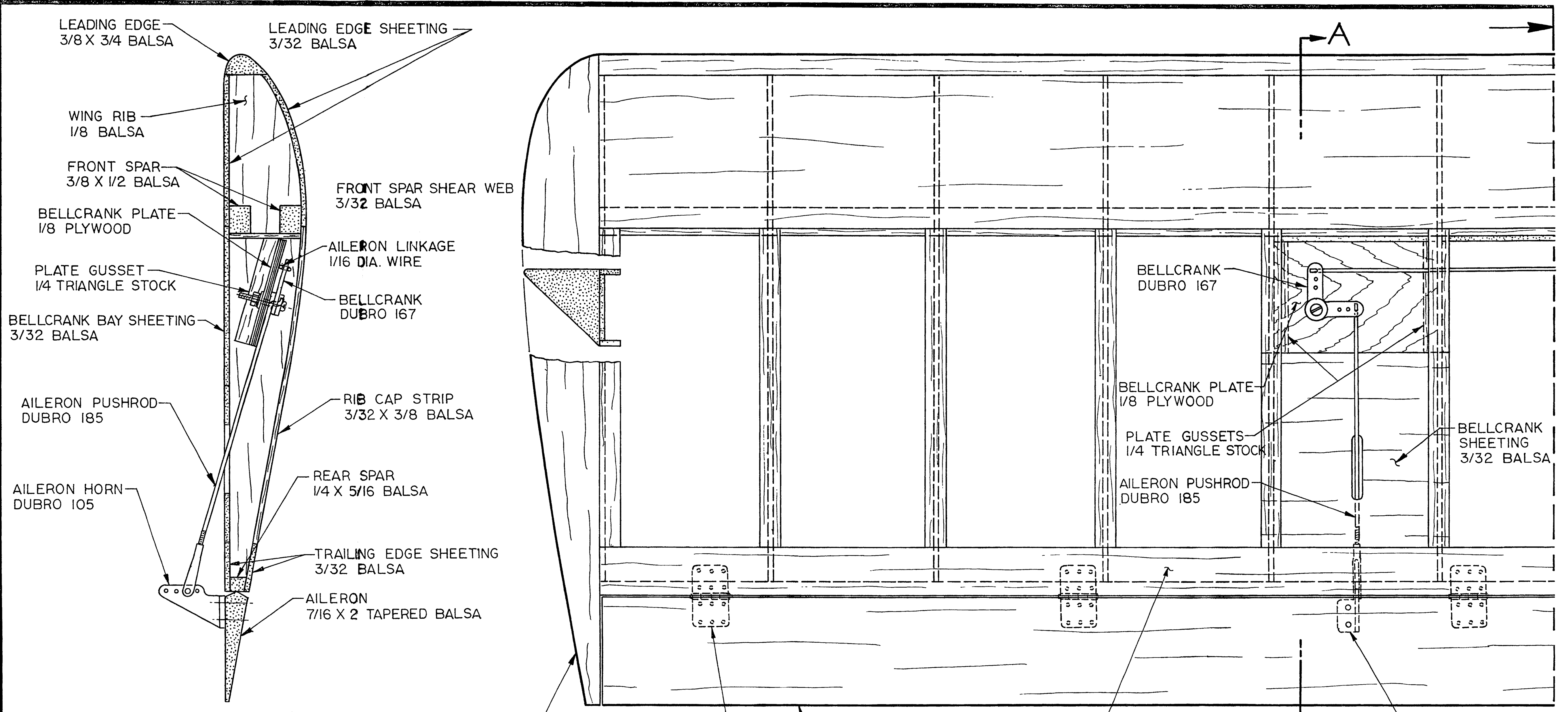
SECTION A-A
