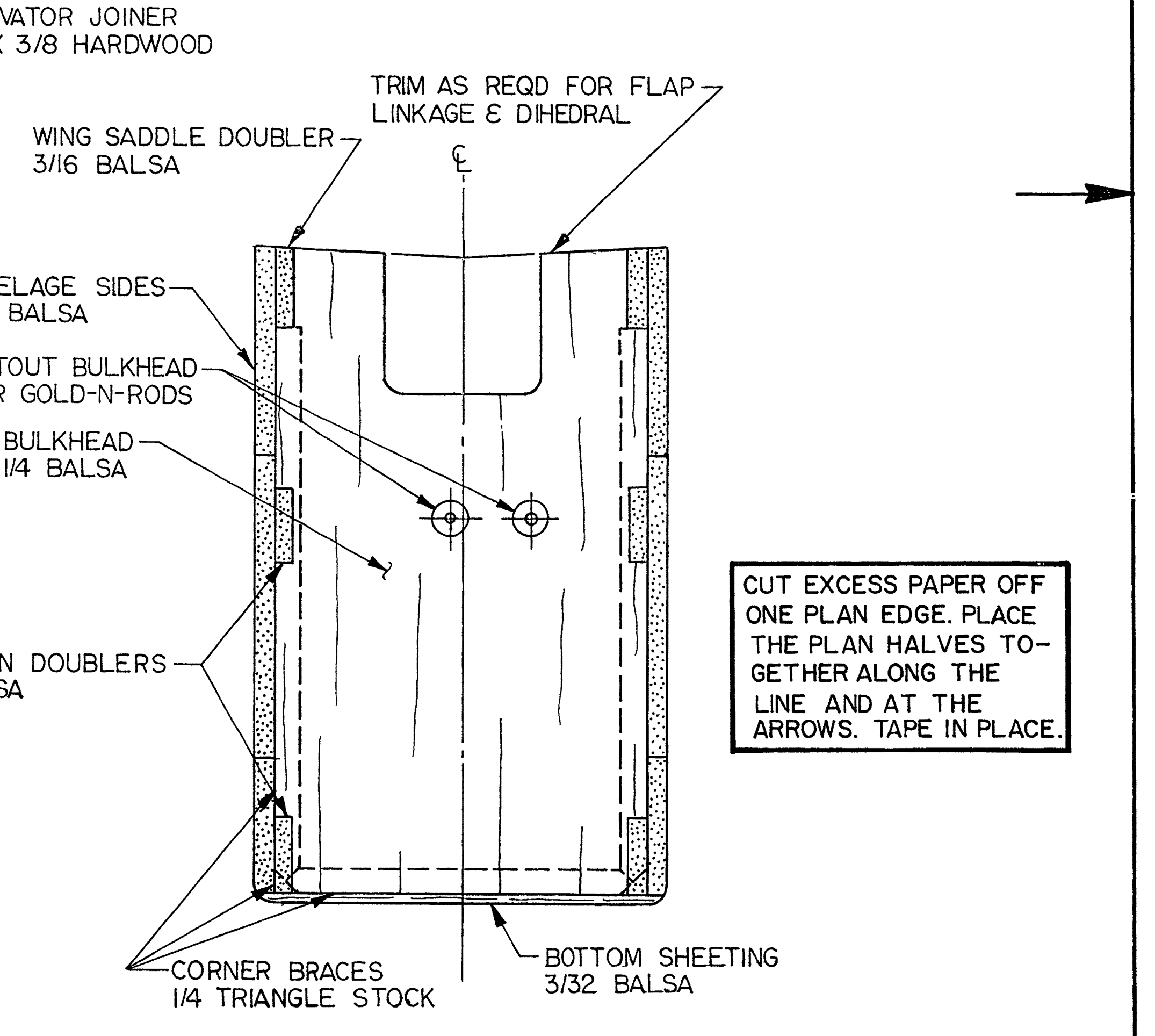
SECTION D-D
