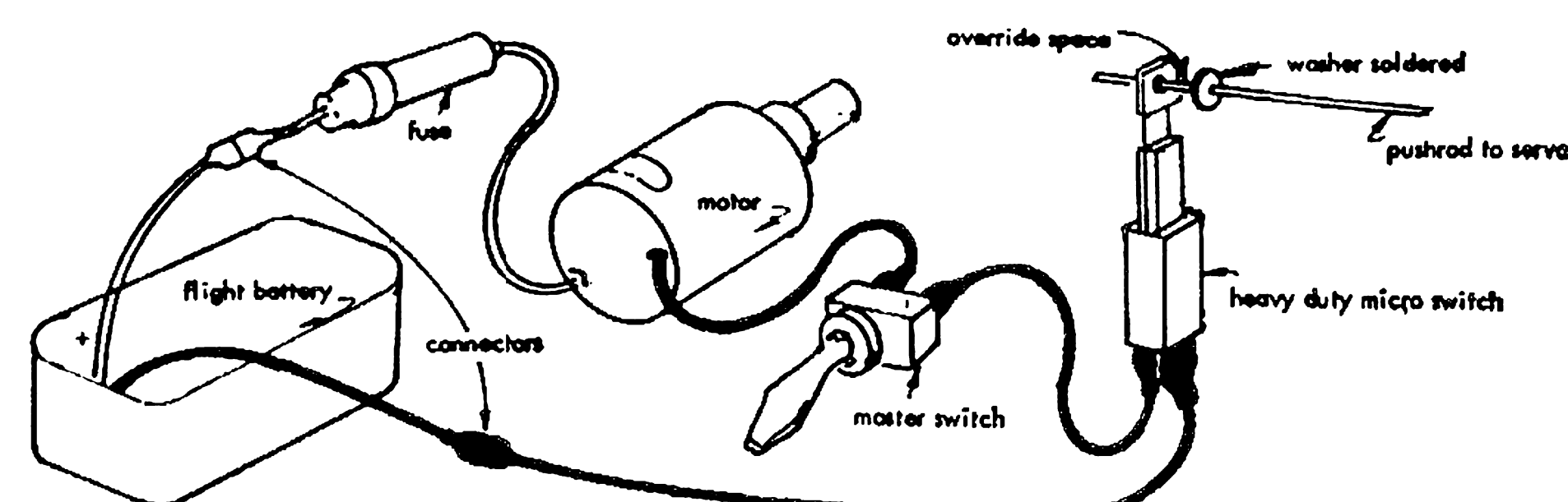
WIRING
