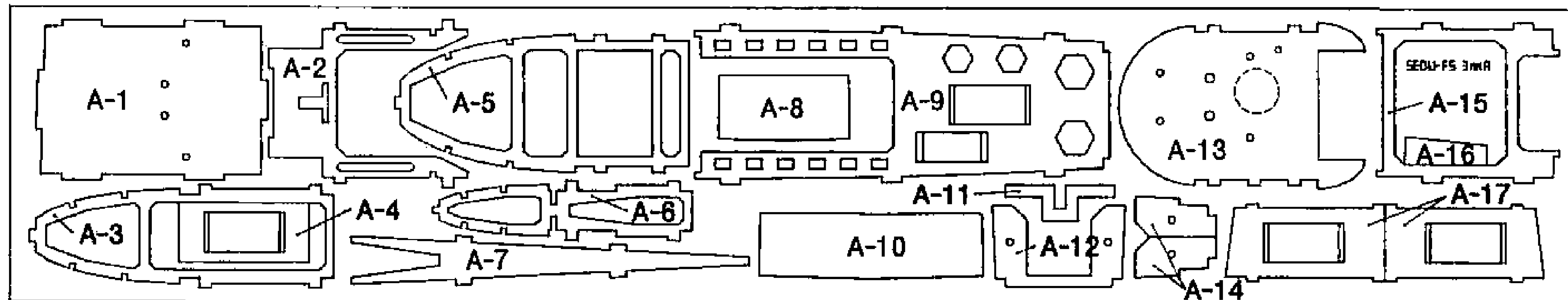
C : 2mmバルサ Balsa X 2
