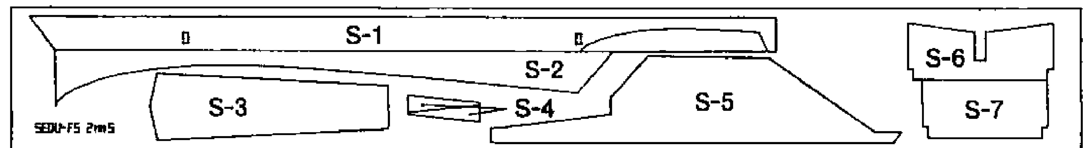
T : 2mmバルサ Balsa
