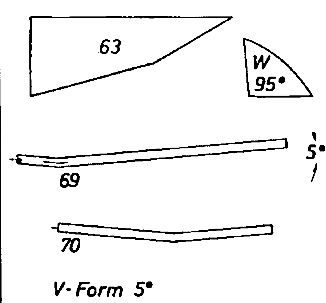
61 53 66 67 Schnitt E-E
