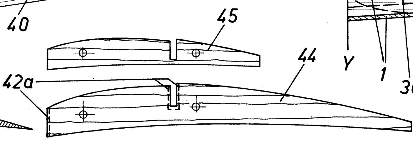
Schnitt B-B
