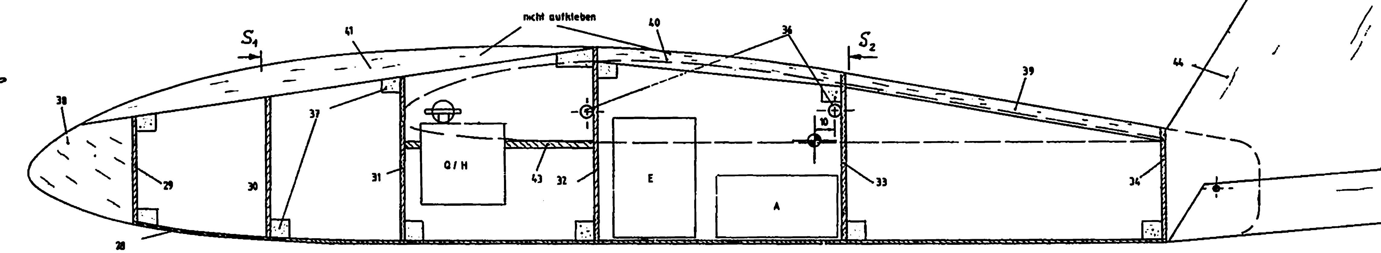
Rumpfaufsicht ohne Haube und Deckel
