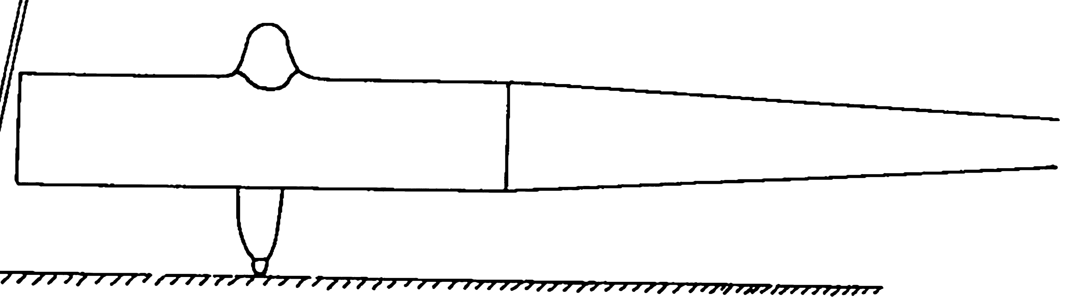
Horten Parabel „Zanonia“ M = 1:15,6
