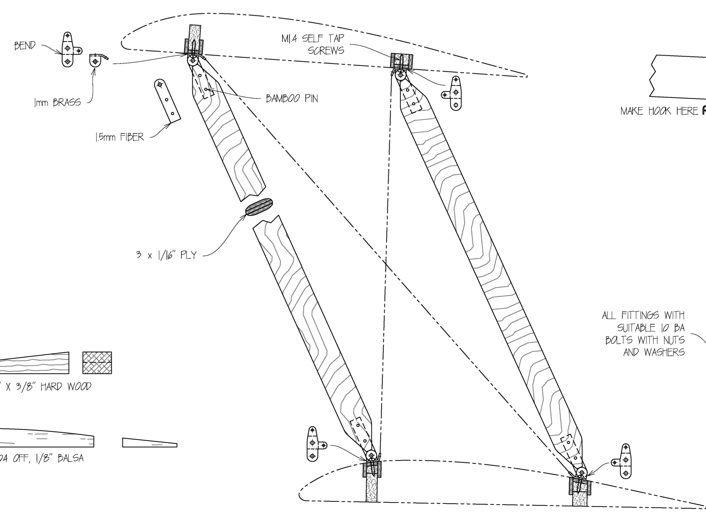
INTERPLANE STRUTS
