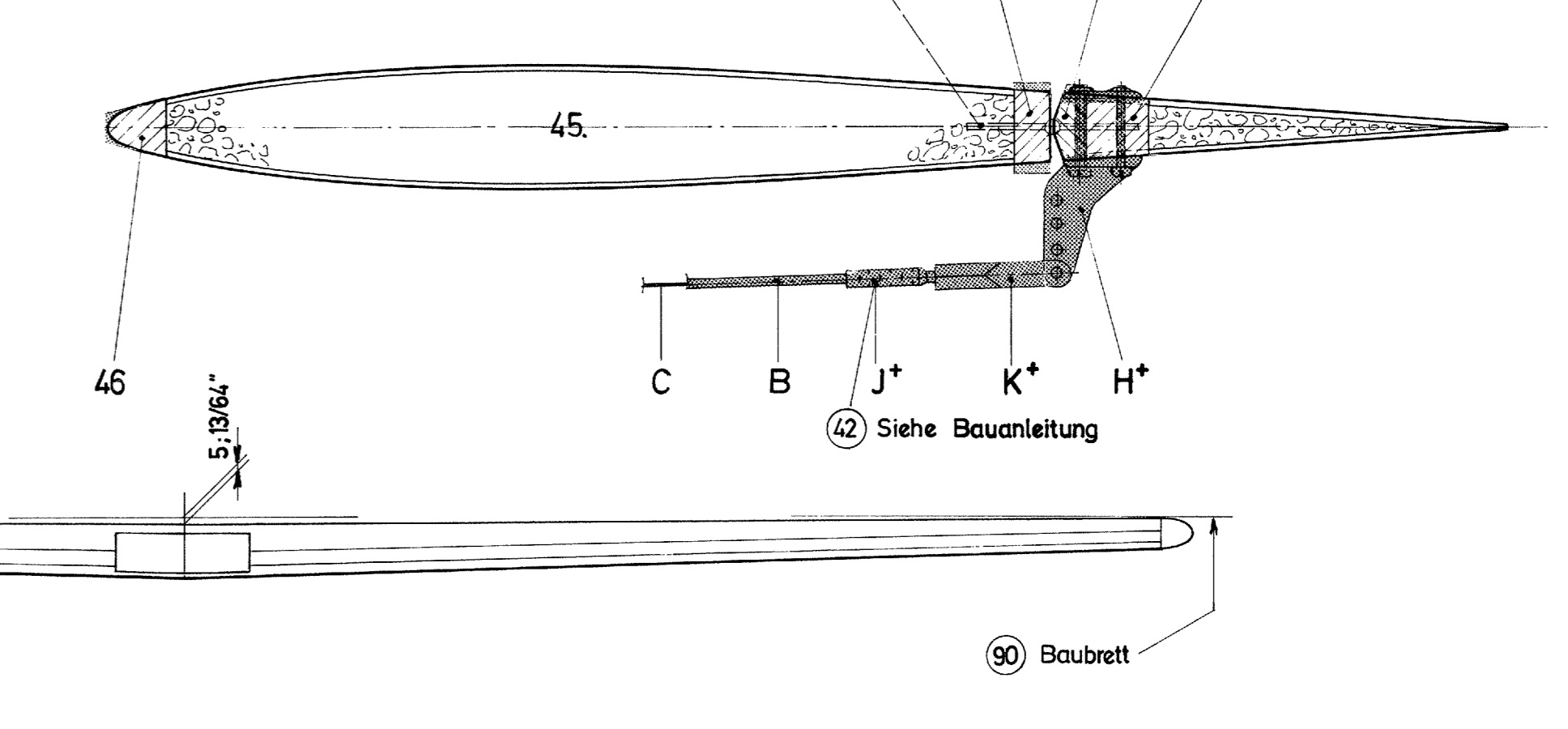
88 Schnitt F-F
