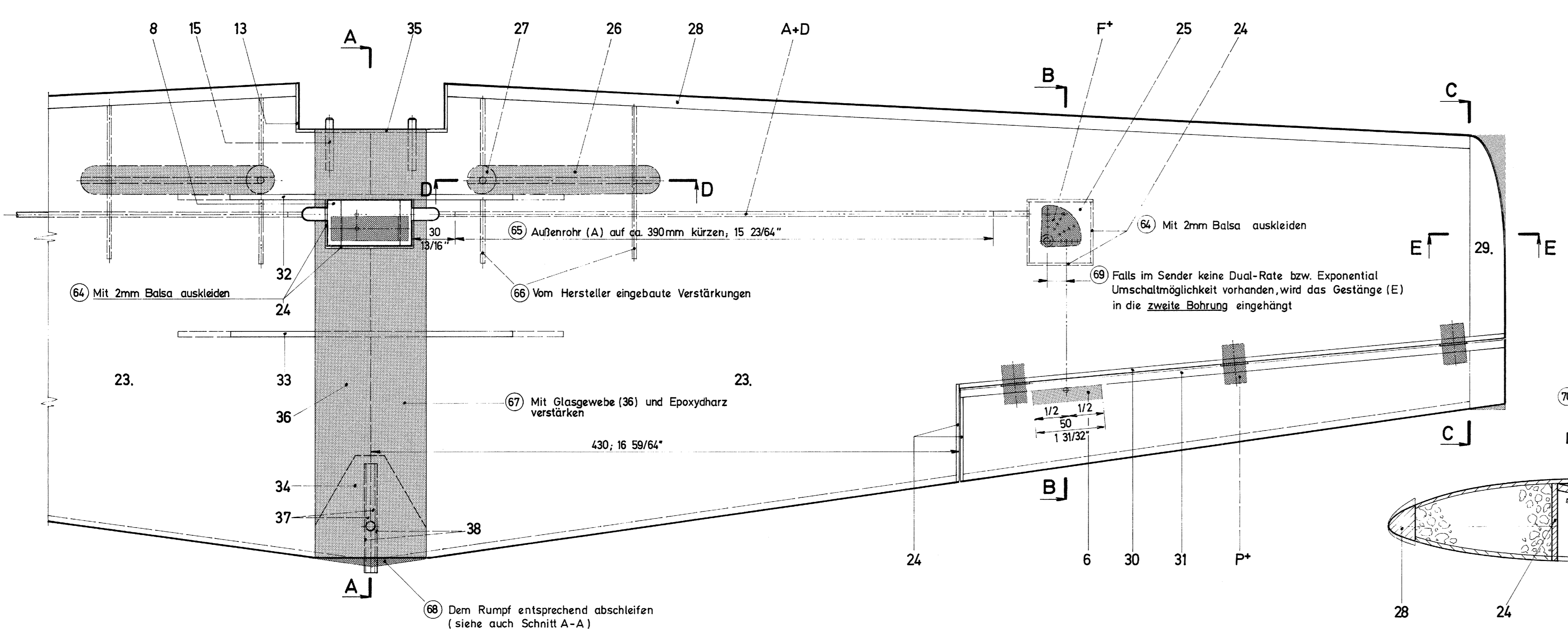
66 FLÜGEL-DRAUFSICHT, M 1:2 (ohne Abschlusspanz (40) und Verkleidung (41) dargestellt)
