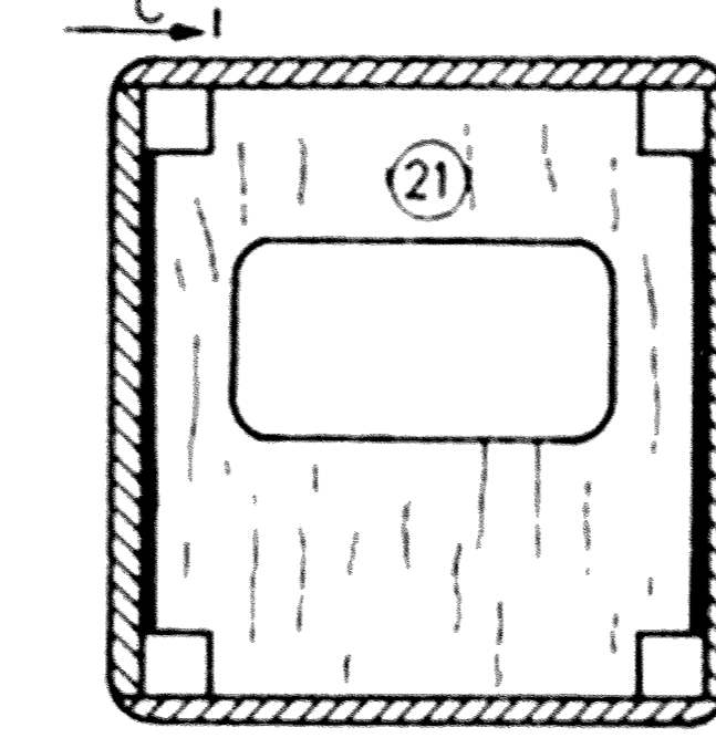
Snit C-C
