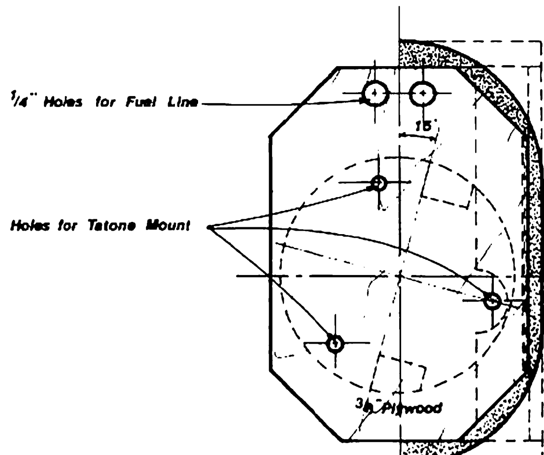
Firewall F1
