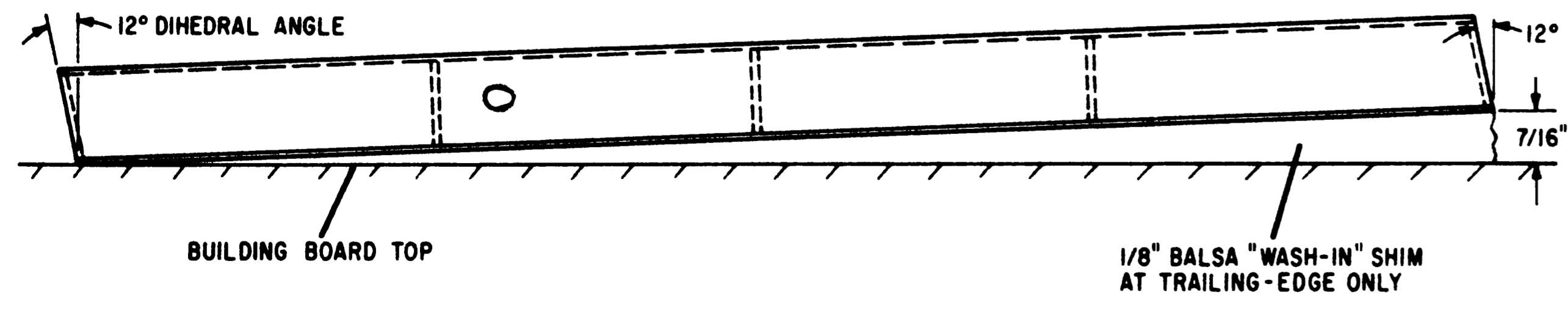
VIEW A-A
